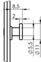
Detail E E ( 1 : 1.5)
